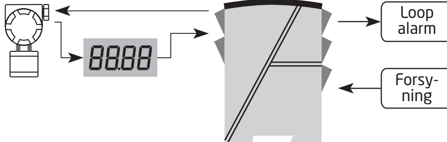
2-Trådstransmitter
