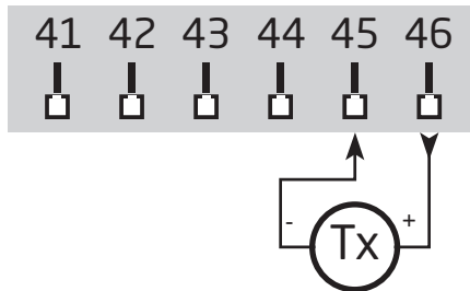
2-trådstransmitter
