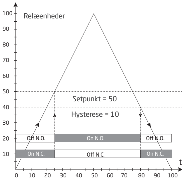
Relæaktion: Stigende
