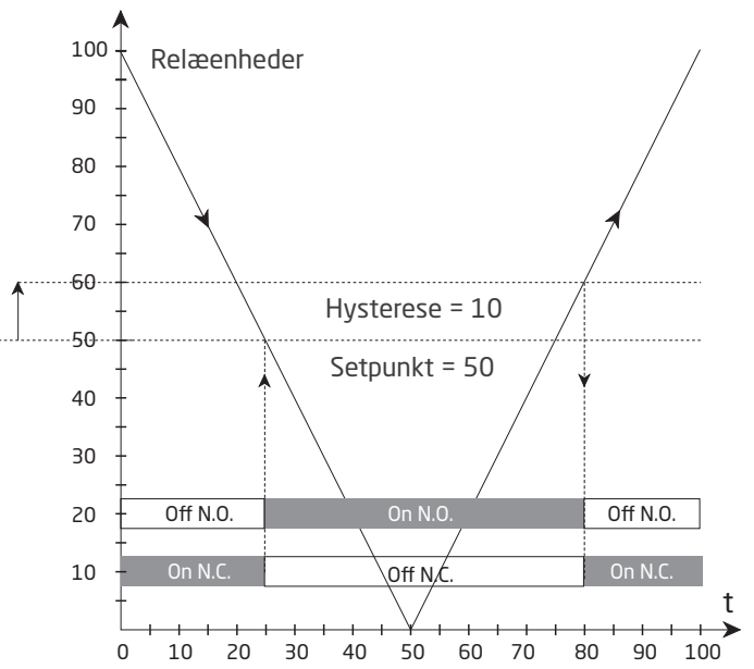
Relæaktion: Faldende
