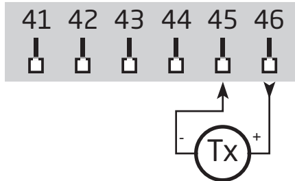
2-trådstransmitter
