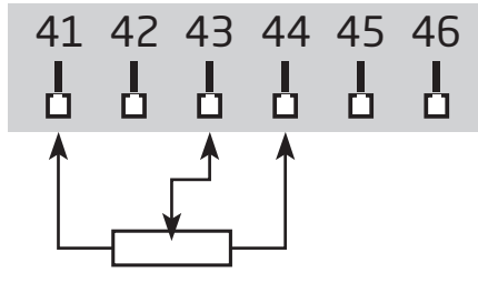
Potenciómetro
