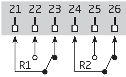
Relés
