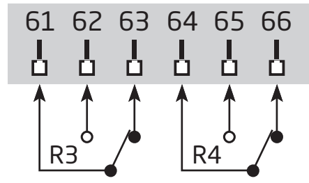
Relés
