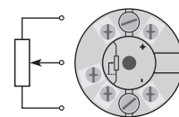
Potentiometer til 4...20 mA
