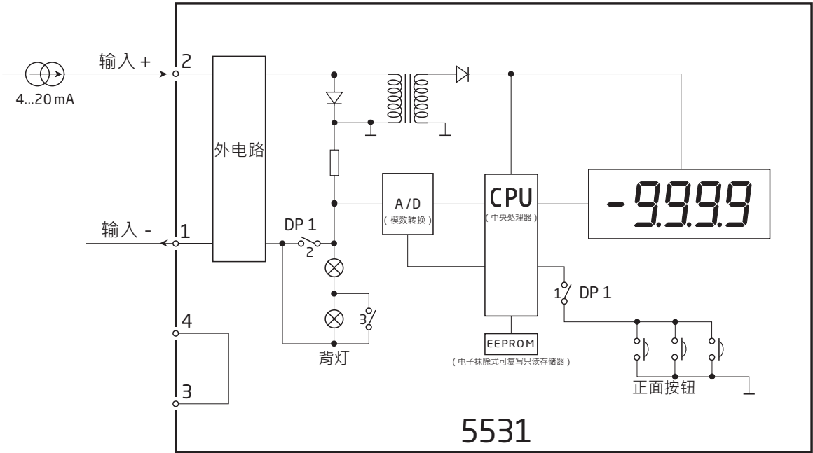
框图
