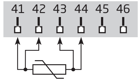
RTD 和线性电阻·4 线制
