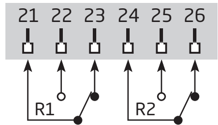
继电器
