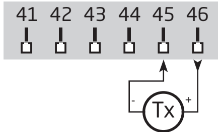
2 线制变送器
