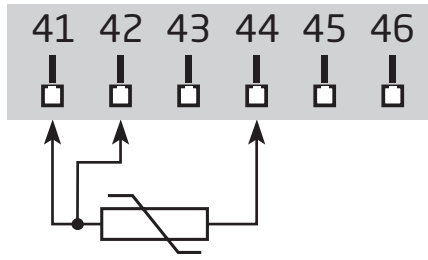
RTD & R Lin, 3-fils
