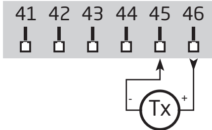
Trasmettitore 2 fili
