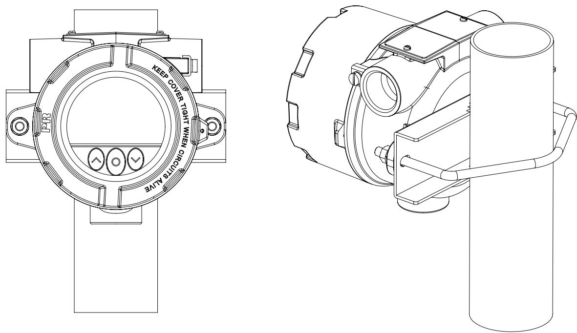
Rohrbefestigung - Draufsicht
