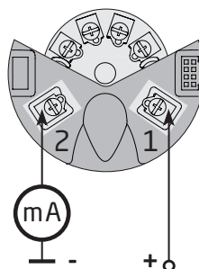
2-проводн. подкл.
