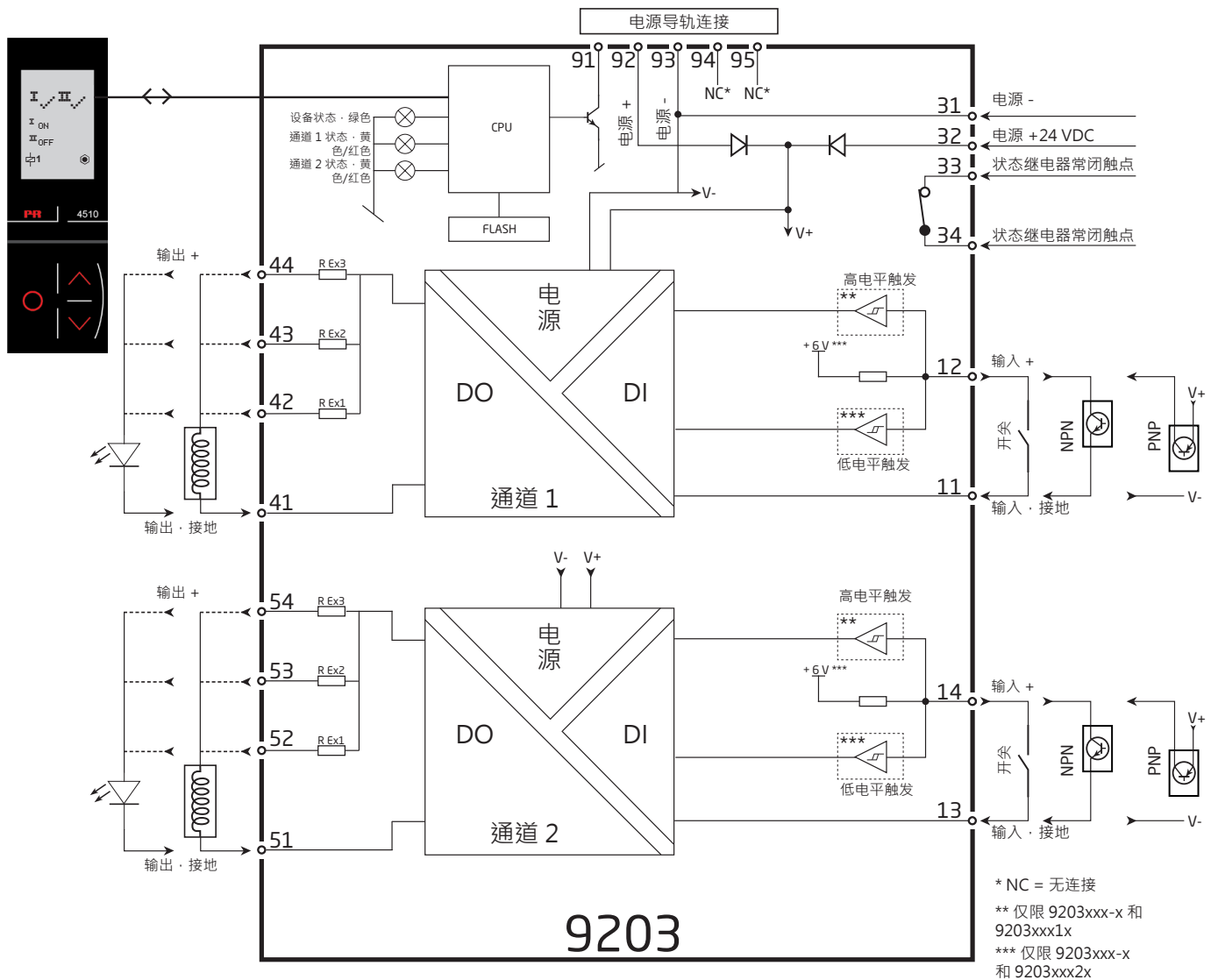
方框图
