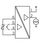
7501 Feltmonteret HART temperaturtransmitter
