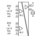
6437A 2-tråds HART temperaturtransmitter
