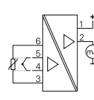
7501 Trasmettitore di temperatura HART con montaggio sul campo
