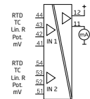
6437A 二线制 HART 7 温度变送器
