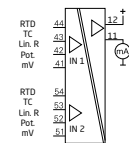
6437D 二线制 HART 7 温度变送器
