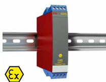
6335D / 6337D 二线制 HART 变送器
