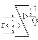
7501 现场安装型 HART 温度 变送器
